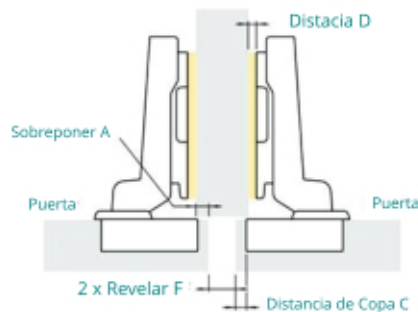
Bisagra Semi Codo (9.5mm acodamiento)
